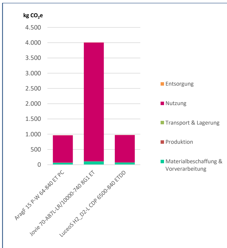
Abbildung 2: Ergebnisübersicht allgemein
